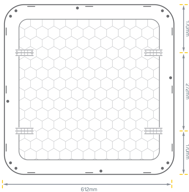
Fig. 3 - Panou ancorare
