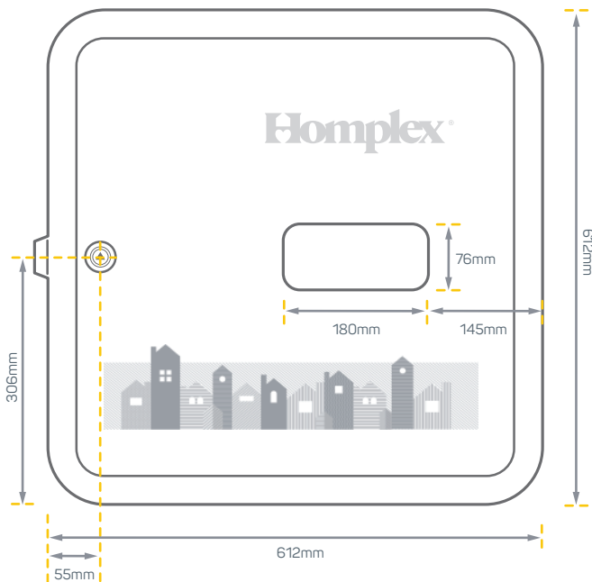
Fig. 3 - Panou ancorare
