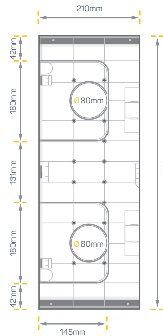
Fig. 4 Perete lateral
