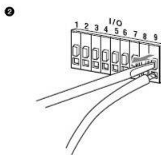
Figura 9-5 Scoateți cablul
