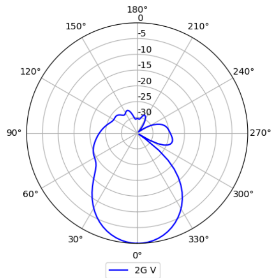
2.4GHz (Vertical)
