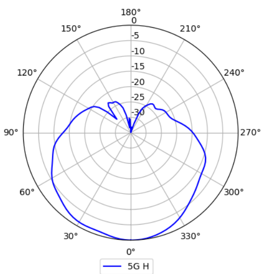
5GHz (Horizontal)
