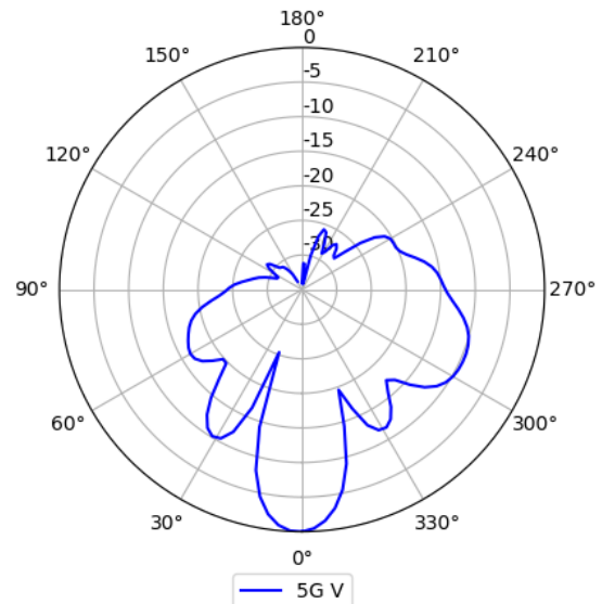
5GHz (Vertical)
