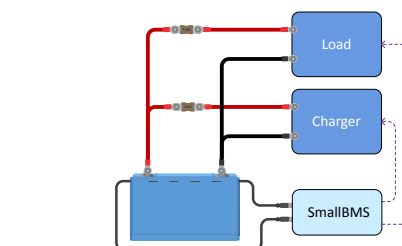
SmallBMS controlează sarcinile și încărcătoarele prin semnale de „deconectare sarcină” și „deconectare încărcare”
