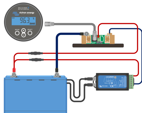
Cablul de alimentare al dispozitivului de monitorizare a bateriei este conectat la baterie
